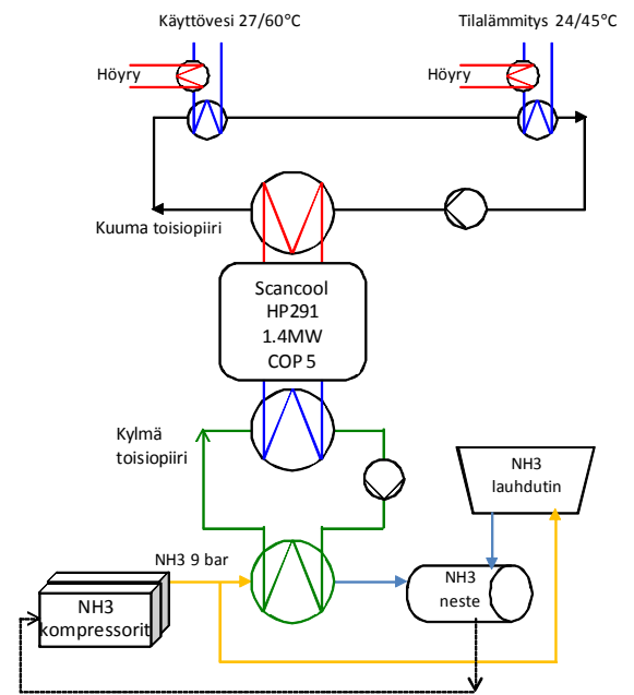
Lämpöpumpujärjestelmän konseptikuva.
