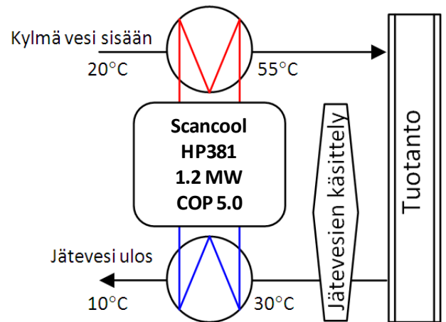
Lämpöpumpun kytkentäperiaate.
