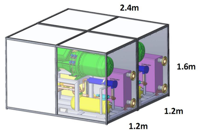
3D-mallikuva kahdesta HP-moduulista suojaseinien kanssa.
